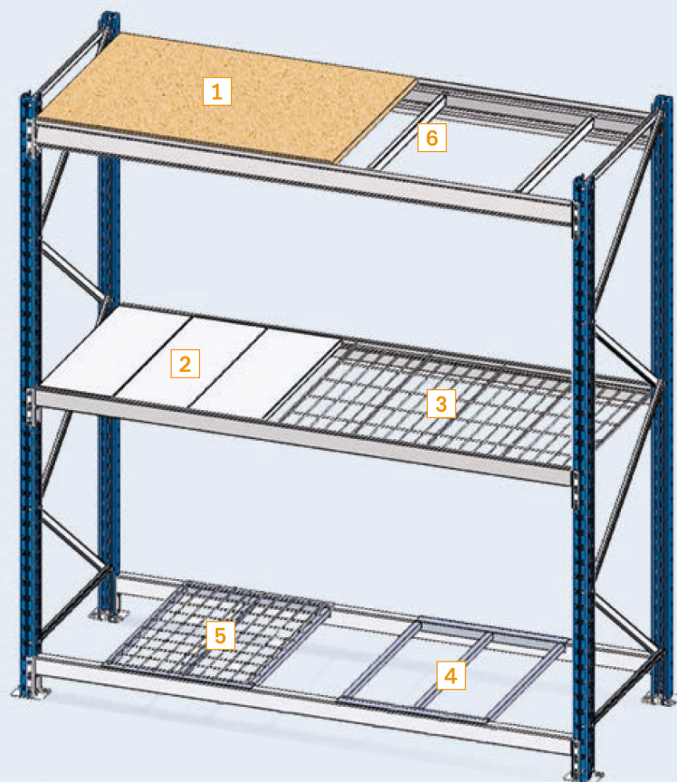
Wit melamine legborden 19 mm
